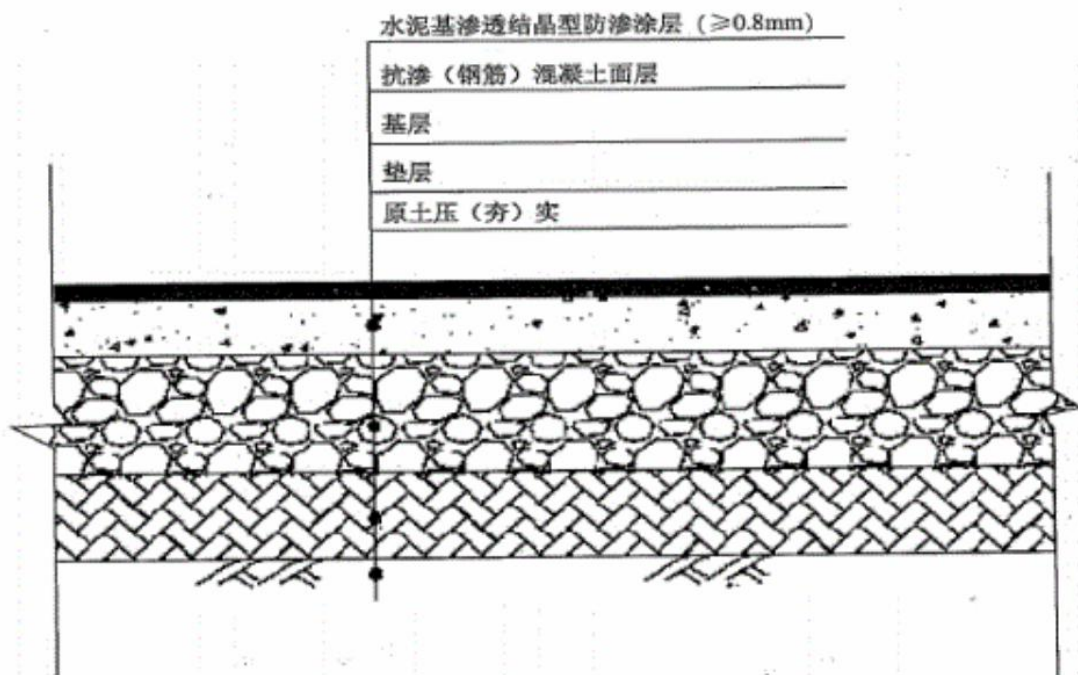
图 7.4-1 地坪防渗层示意图
