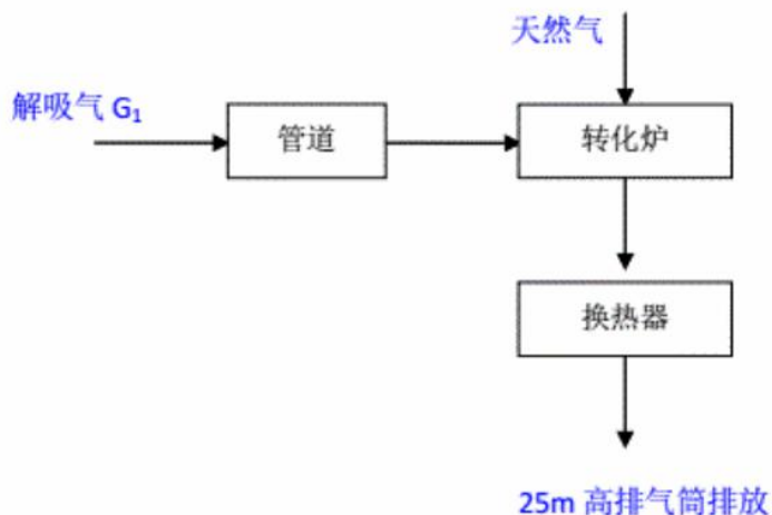
图 7.1-1 全厂废气收集、处理流程图
