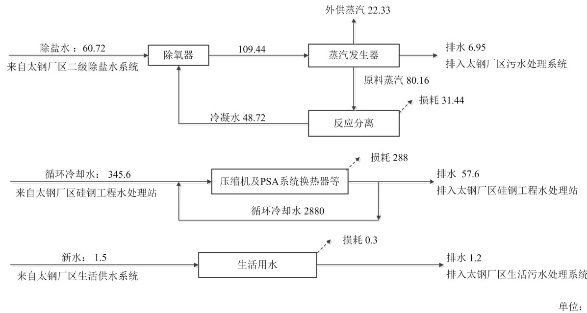
图 3.1-2 项目水平衡图
