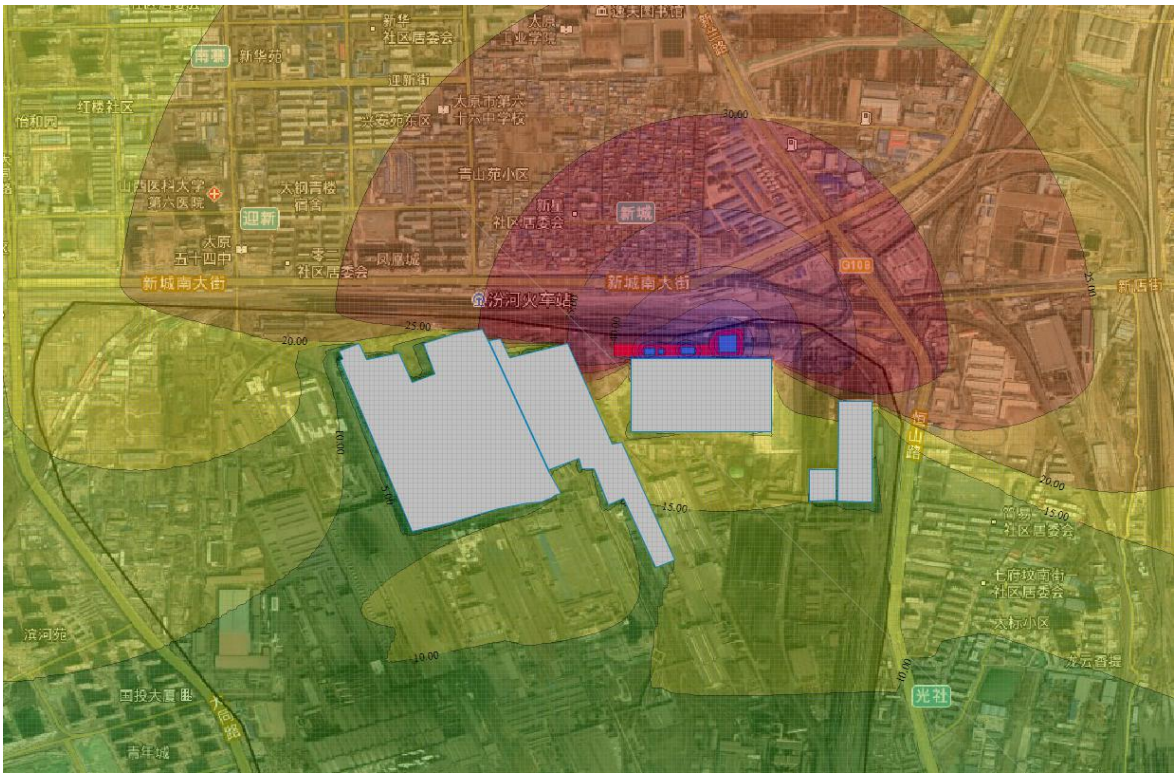
图 5.5-2 项目噪声预测等值线图
