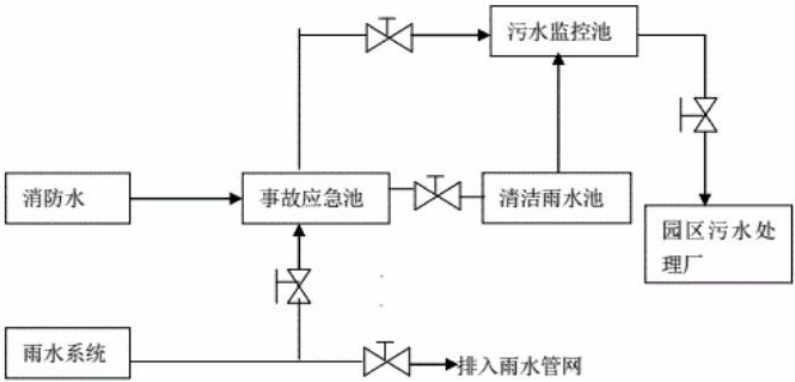
图 6.6-2 事故状态下厂区排水与外部水体的切断措施示意图
