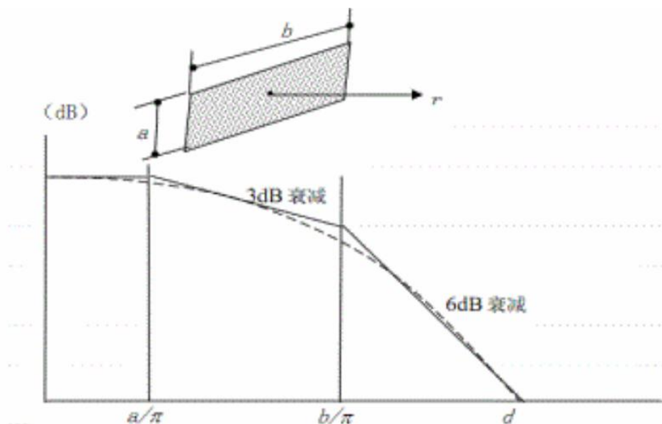
图 5.5-1 长方形面声源中心轴线上的衰减特性
