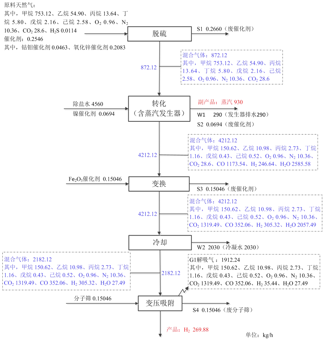
图 3.1-1 建设项目原料天然气部分物质平衡图
