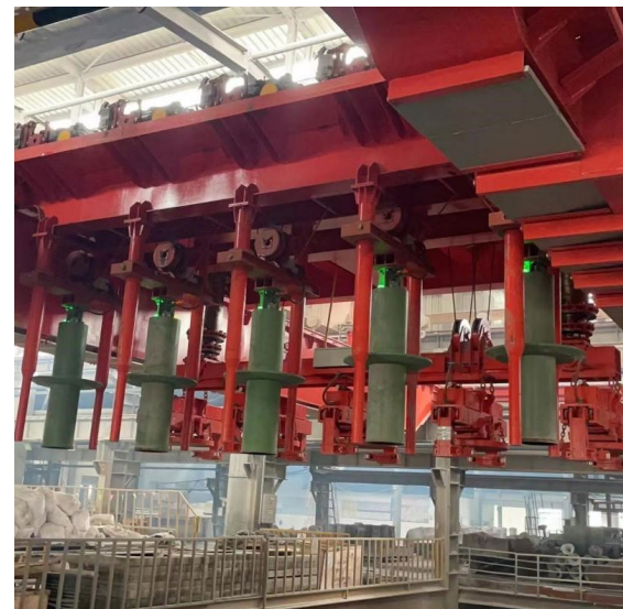
重载桁架机器人
