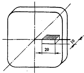
图 A2 非金属夹杂物取样方法
