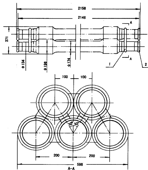
图 B2 车轴包装方法示意图
